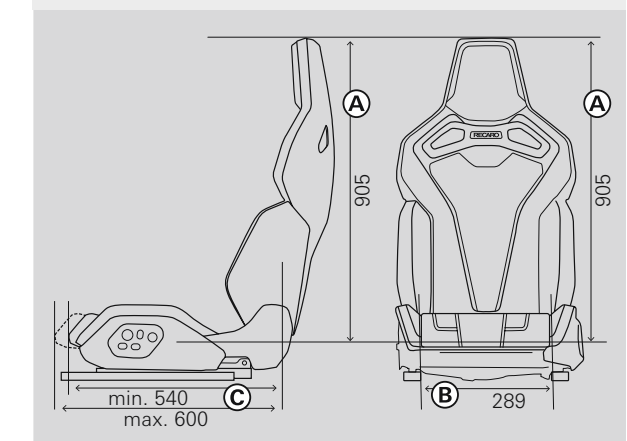
A: Sitzhöhe | B: Sitzbreite | C: Sitztiefe Maße in mm, alle Angaben +/- 10 mm
